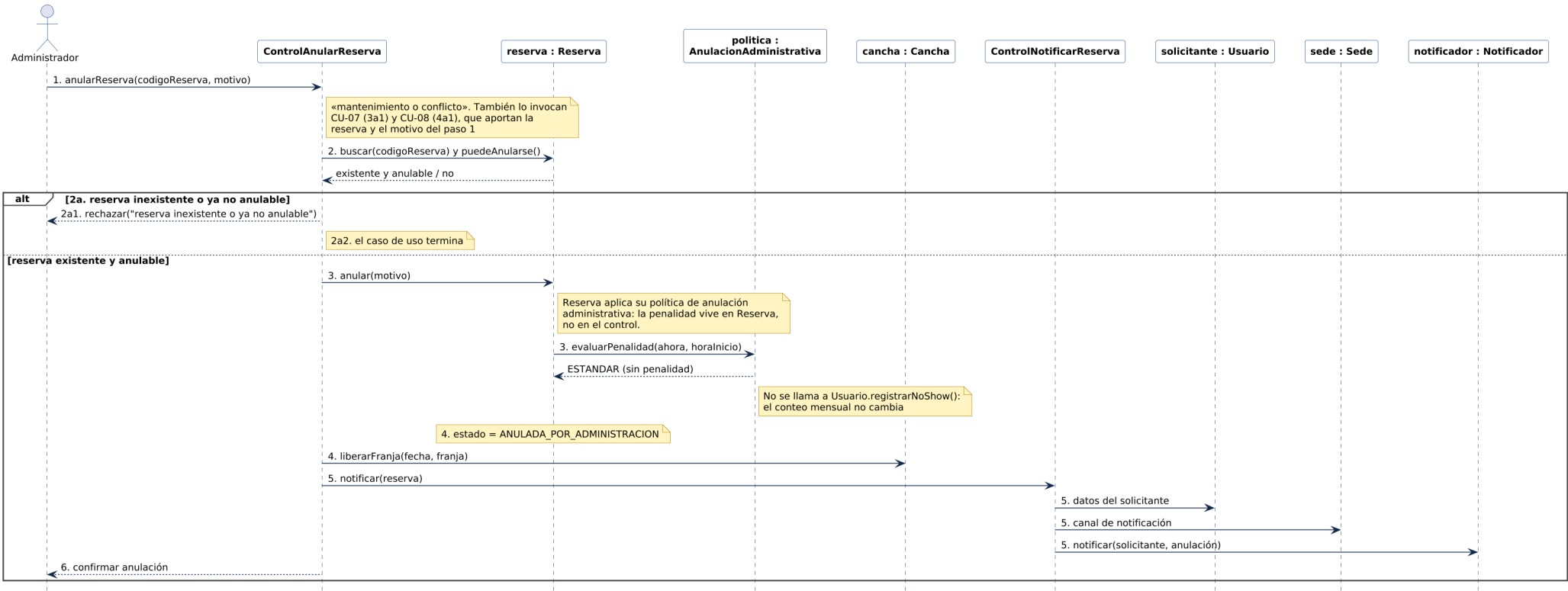
Secuencia: Anular Reserva sin Penalidad (CU-09)
